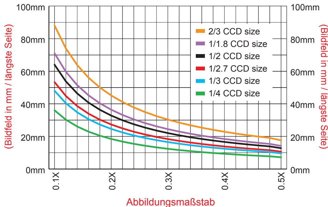
Zusammenhang zwischen Abbildungsmaßstab und Bildfeld
