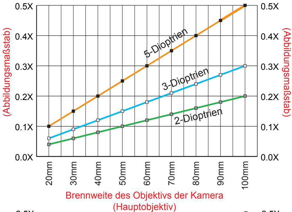
Zusammenhang zwischen Dioptrien und Abbildungsmaßstab
